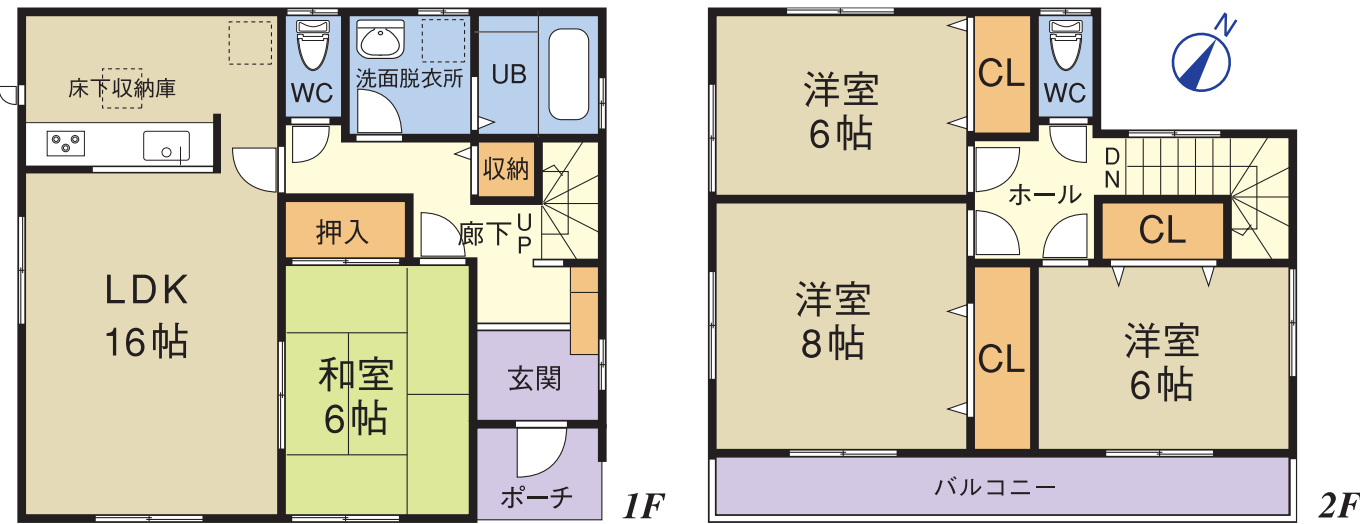
1号棟間取図
