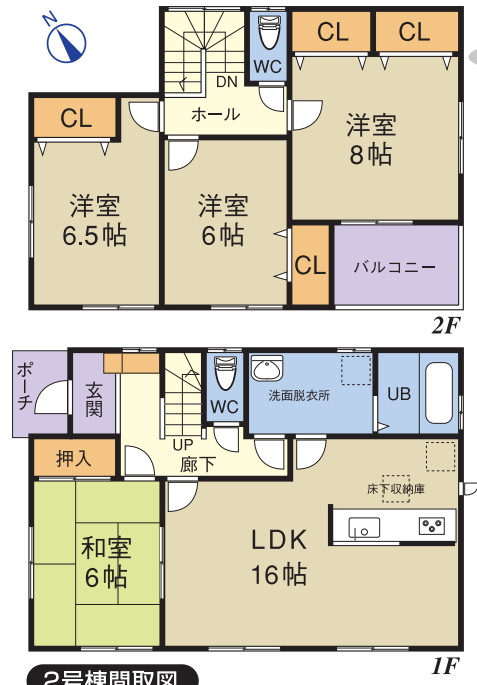
2号棟間取図
