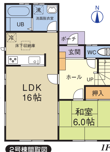
2号棟間取図
