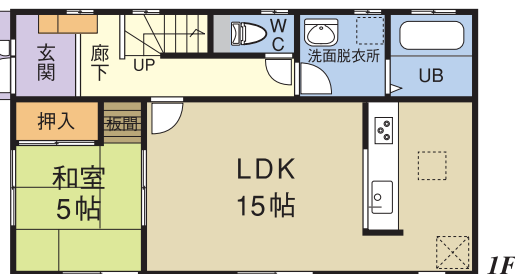
3号棟間取図
