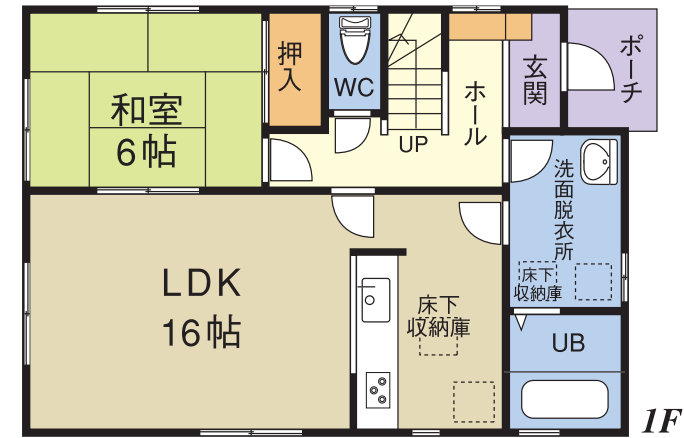
2号棟間取図
