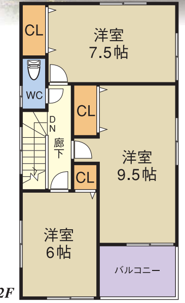
1号棟間取図
