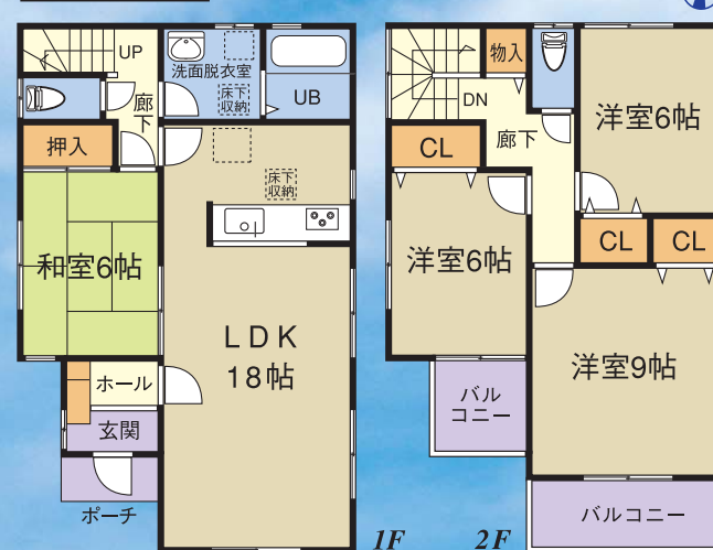
1号棟間取図
