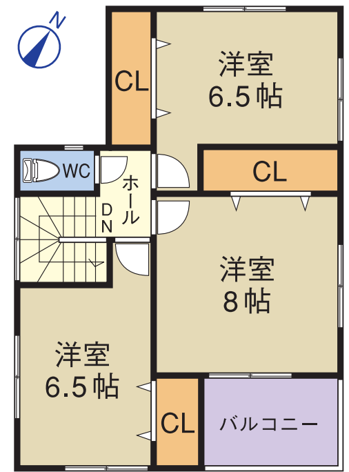
2号棟間取図
